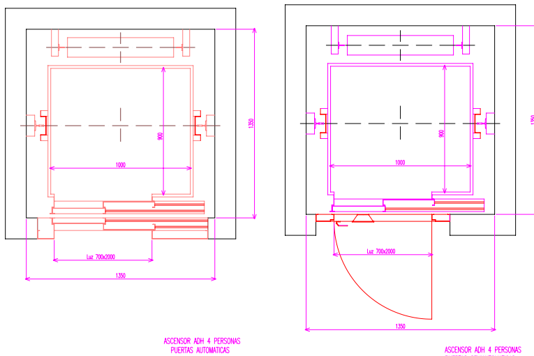
Esquema de montaje de ascensor
