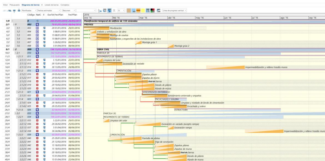
Planificación de edificio de viviendas: barras ASAP, ALAP y holguras
